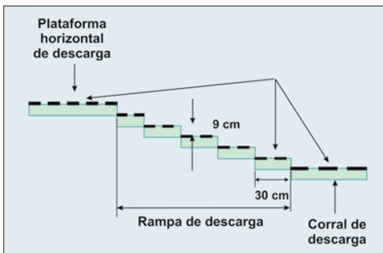
Diseño de rampas de carga y descarga de animales.
