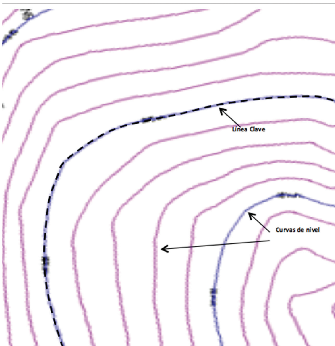
Figura 7. Predio con curvas a nivel y Línea Clave.
