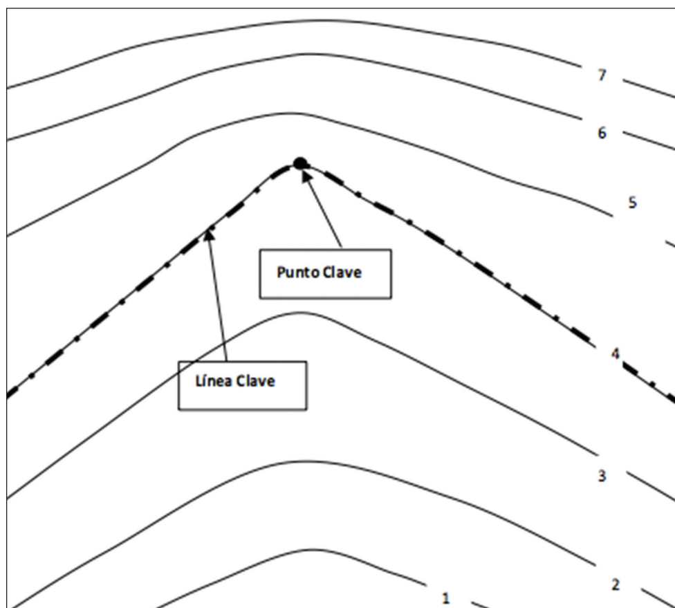
Figura 3. Plano de curvas a nivel identificando la Línea Clave.
