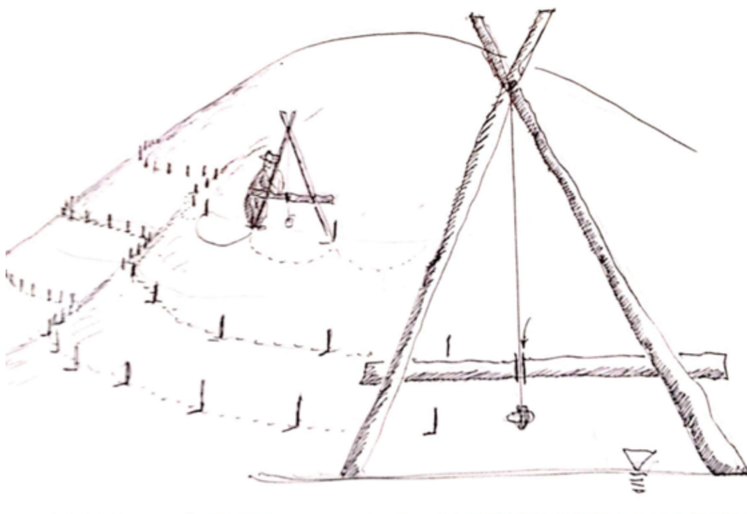
Figura 9. Forma de obtener curvas de nivel en el terreno con el nivel "A".
