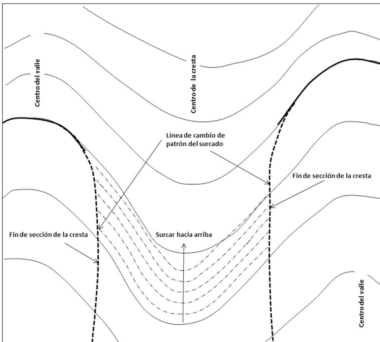
Figura 16. Predio donde se muestra la línea frontera entre cresta y valle, e inicio del surcado.
