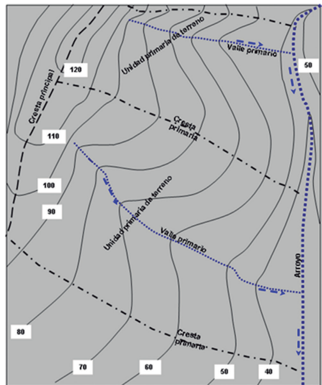
Figura 1. Plano de curvas a nivel que identifican crestas y valles.
