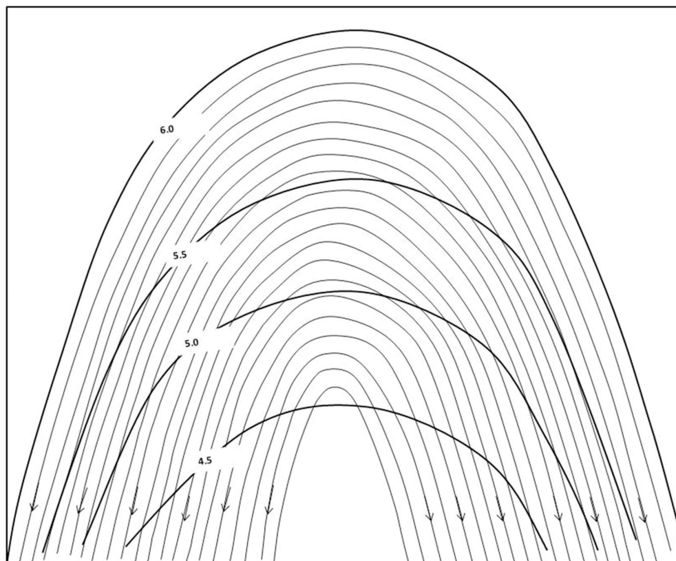
Figura 15. Predio en un valle. El surcado envía el agua hacia sus lados, rumbo a la cresta.
