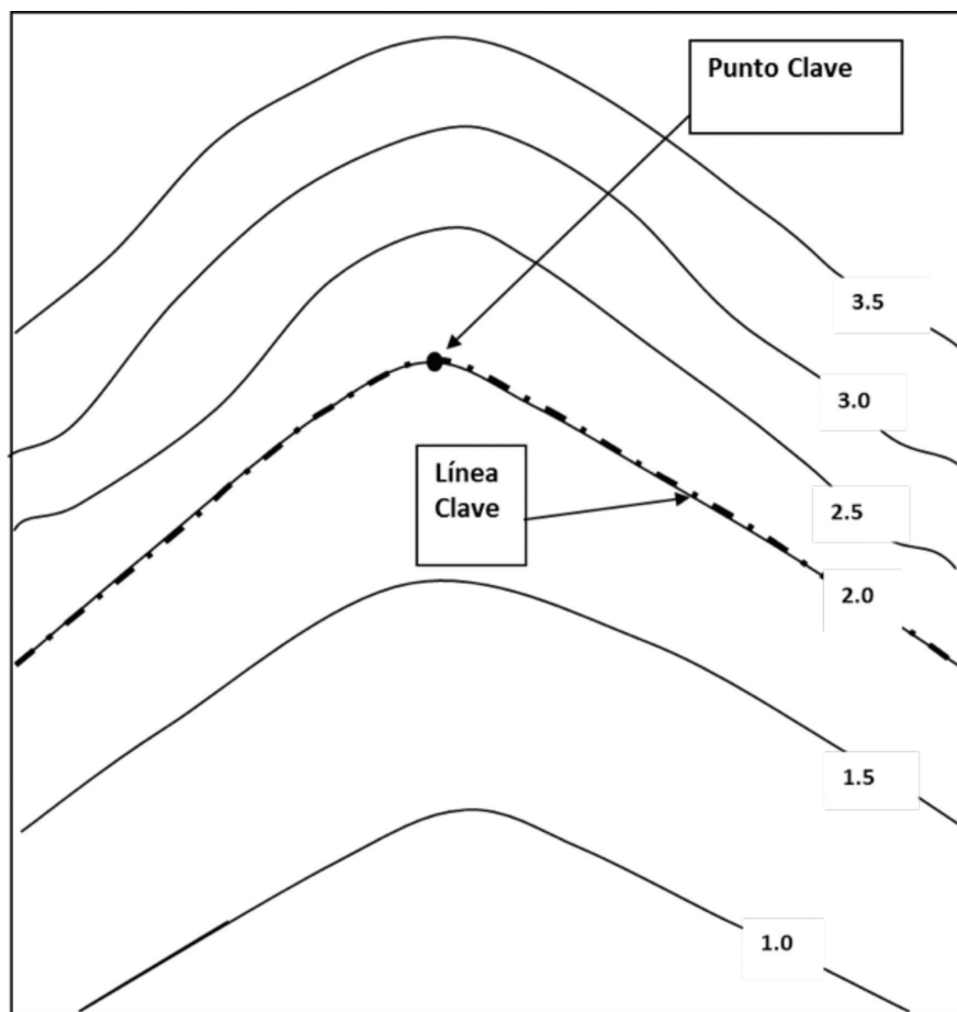
Figura 4. Localización del Punto Clave y Línea Clave en el plano de una parcela.
