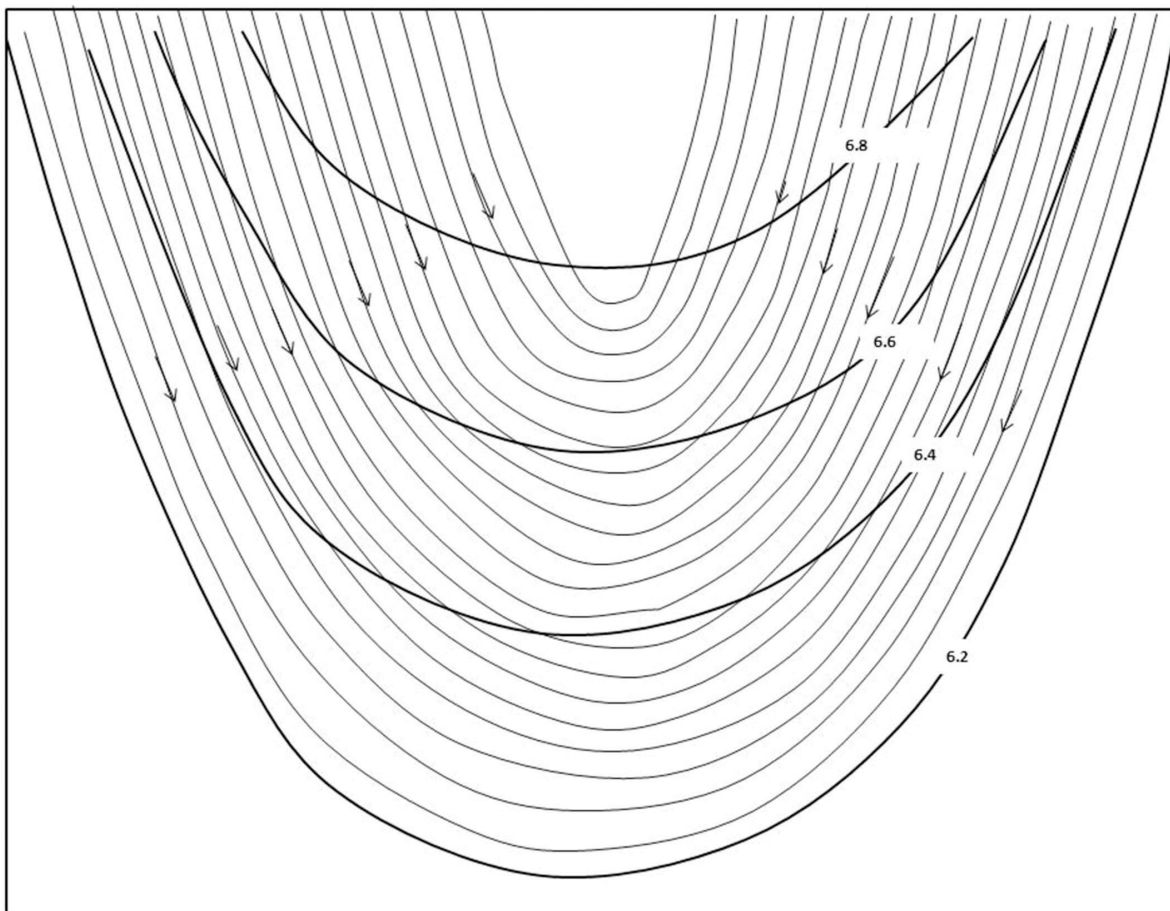
Figura 14. Predio en una cresta o lomo. El surcado envía el agua hacia la cresta.
