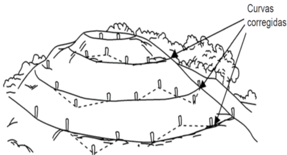
Figura 10. Suavizando las curvas de nivel.
