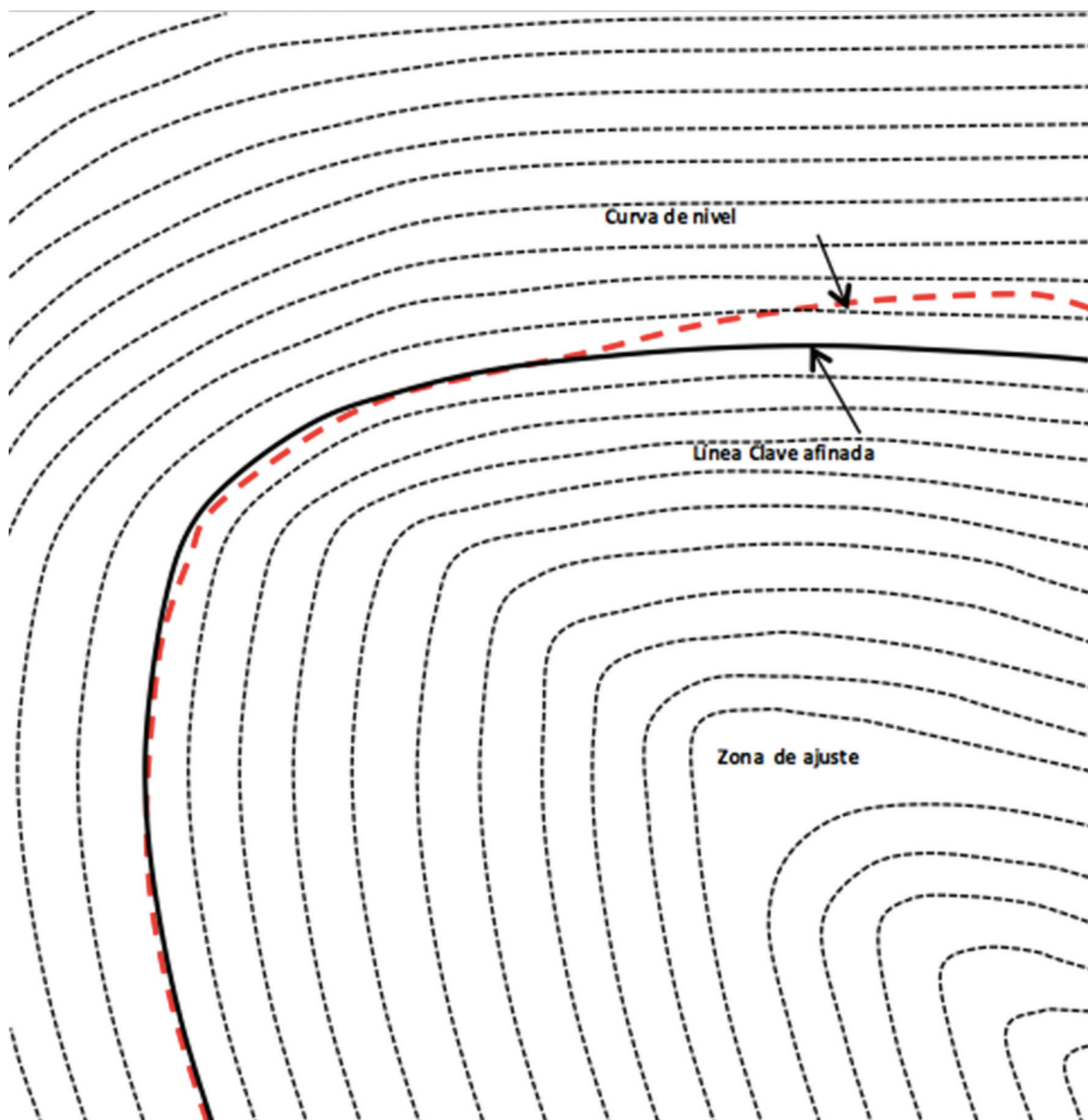
Figura 8. Predio con surcado en Línea Clave.
