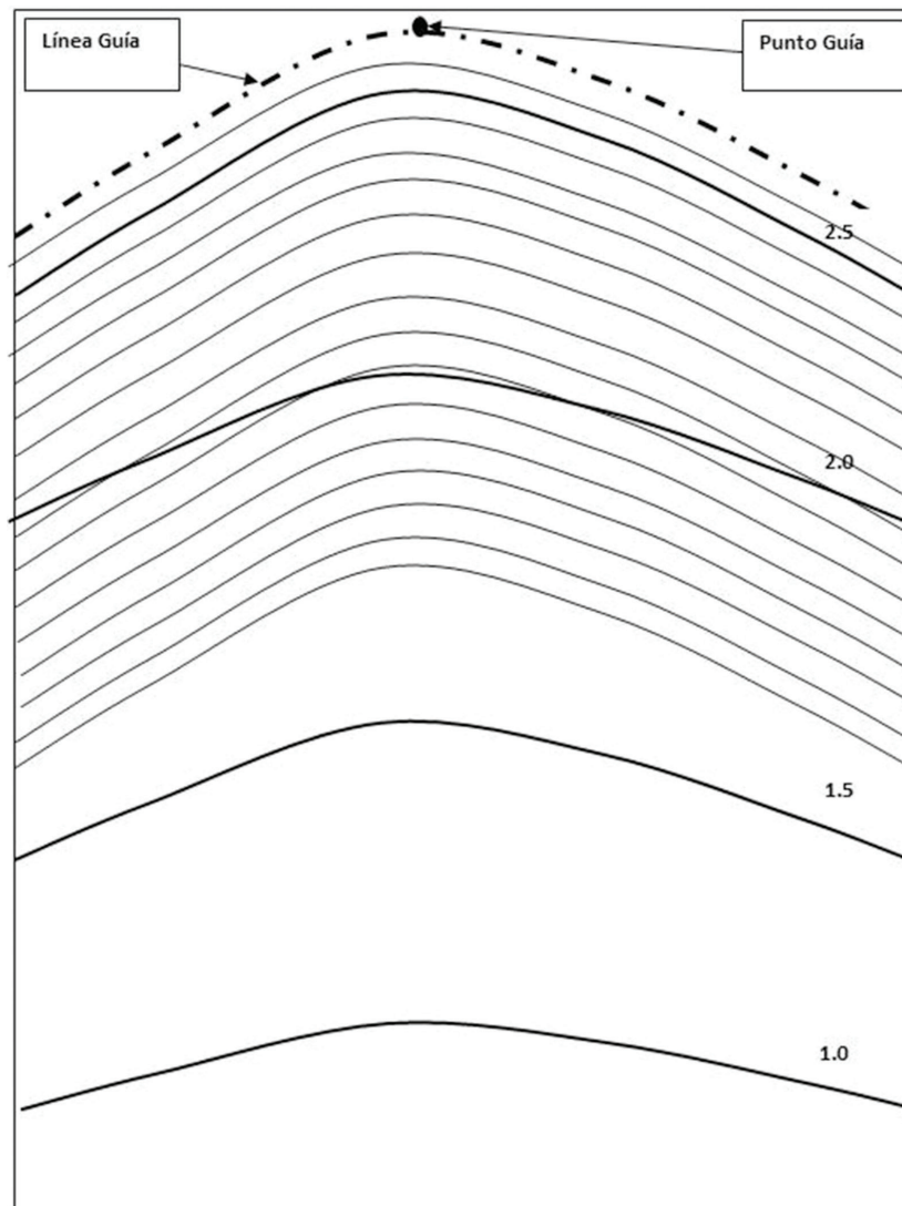
Figura 13. Predio en un terreno muy plano. El surcado envía el agua hacia las crestas.
