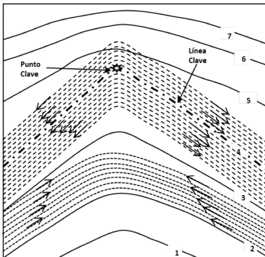
Figura 6. Suroado en línea clave (arriba) y en curvas a nivel (abajo).
