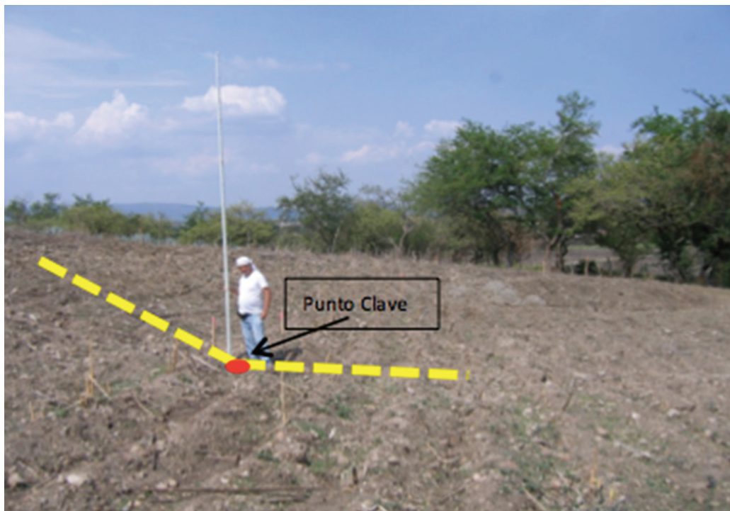
Fotografía 4. Identificación del Punto Clave en el terreno (cambio de pendiente).
