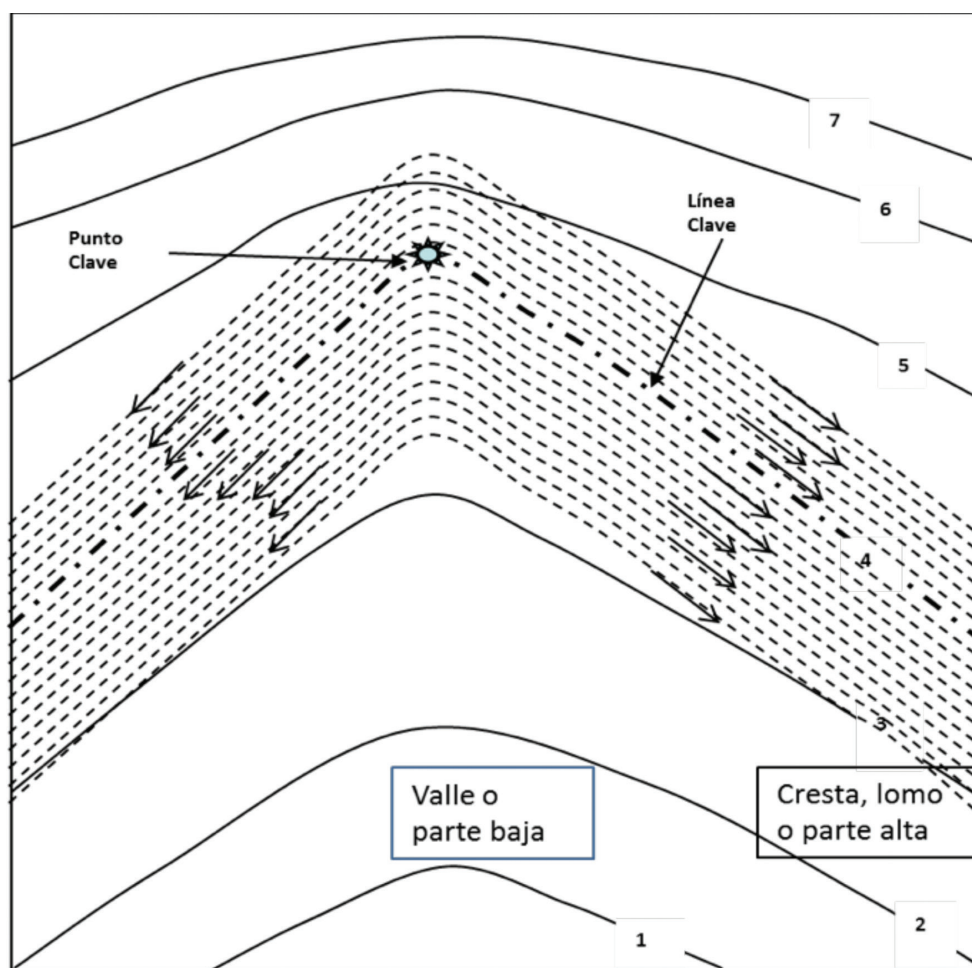
Figura 5. Diseño del surcado en Línea Clave.
