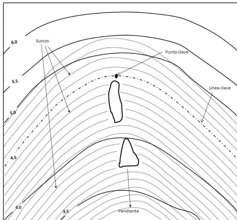
Figura 18. Forma de surcar en un predio en un valle con hoyos en parte baja.
