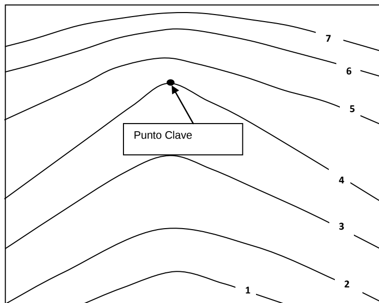
Figura 2. Mapa de curvas a nivel identificando el Punto Clave.
