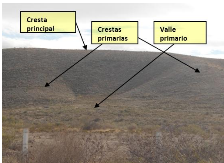
Fotografía 1. Crestas y valles en el paisaje del terreno.
